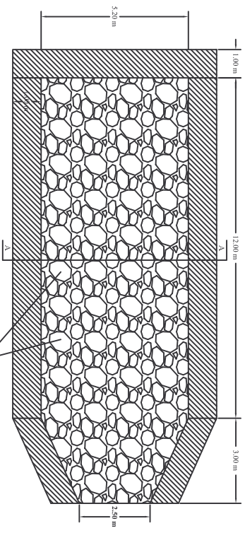
VASCA DI CALMA: Pianta Tipo
